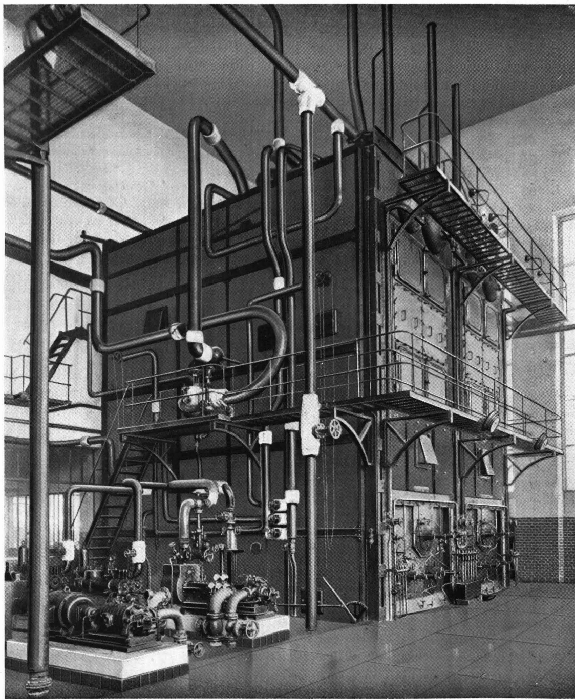
Gruppo caldaie: Tubazioni isolate con « Martinite »
